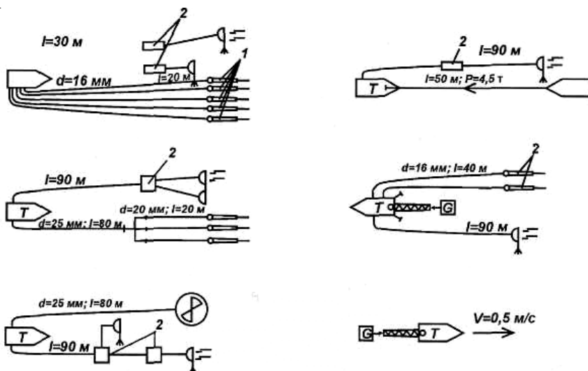
Рис. 7.2. Схемы боевого использования автомобилей технической службы:
