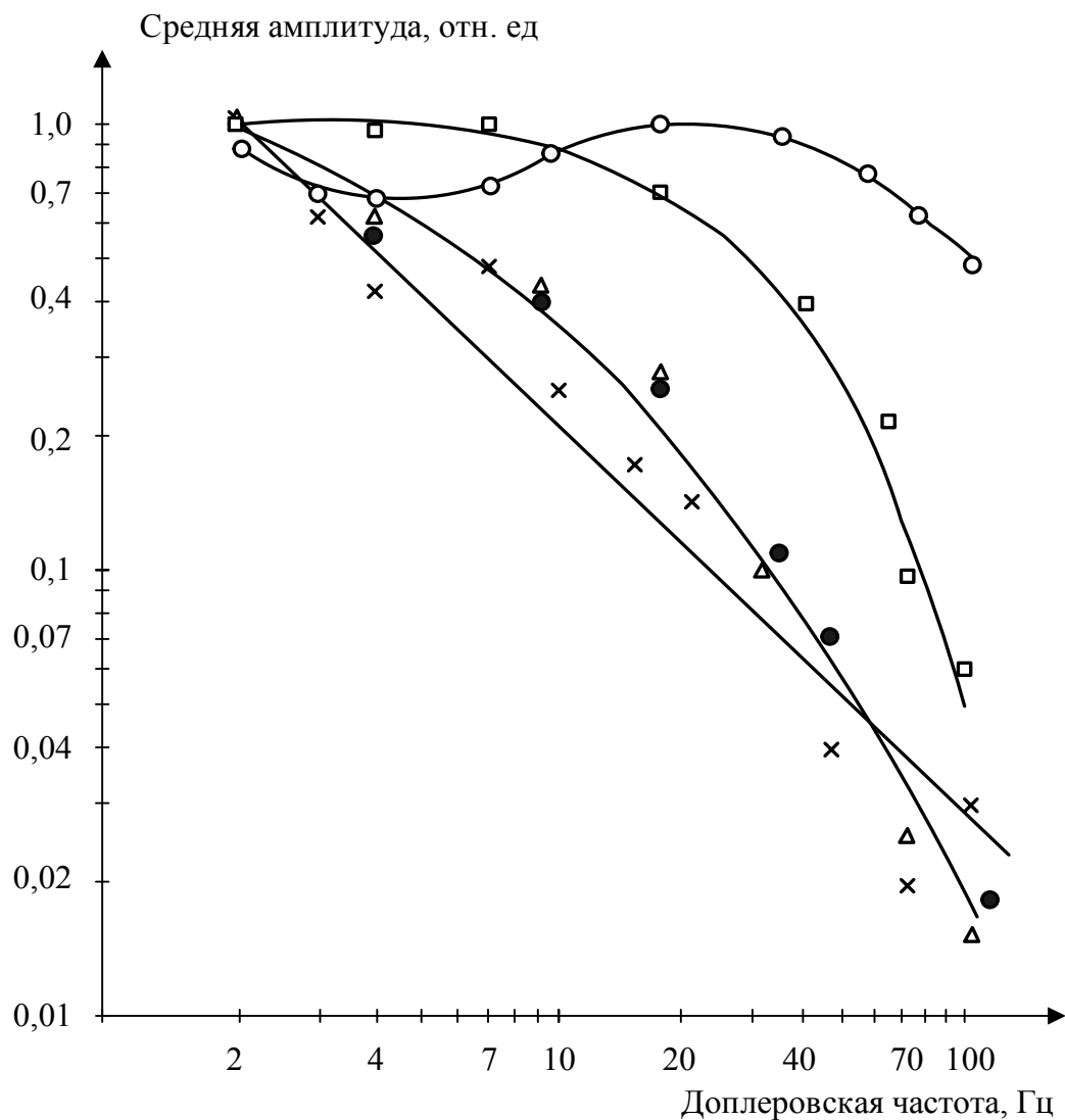
Рис. 1.6. Спектральная характеристика сигналов цели и характерных помех доплеровского извещателя:
