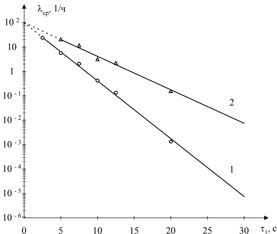
Рис. 5.4. Экспериментальные зависимости интенсивности перемещений людей в помещении с установленной длительностью \tau_1 : 1 – движение человека в одну сторону (на извещатель); 2 – движение человека в любую сторону
