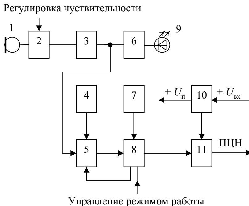
Рис. 5.6. Функциональная схема инфразвукового извещателя:
