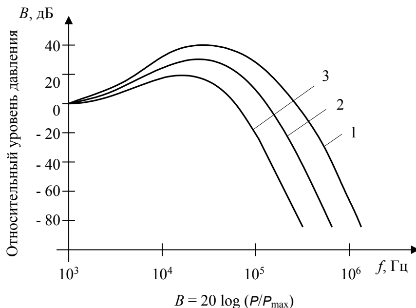
Рис. 5.7. Зависимость формы спектра акустической эмиссии, вызванной терморазрушением, от расстояния до источника: 1 – расстояние 1 м; 2 – расстояние 3 м; 3 – расстояние 6 м
