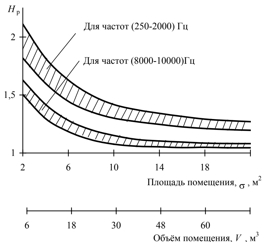
Рис. 5.8. Зависимость относительного времени реверберации от площади (объёма) помещения при измерении в различных диапазонах частот
