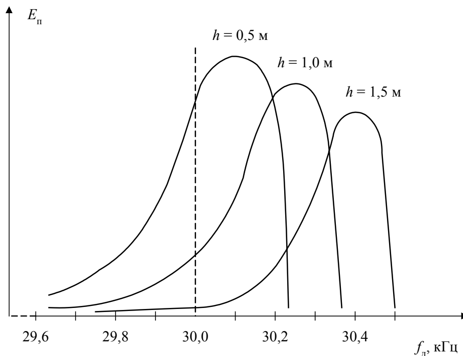
Рис. 5.3. Энергетический спектр сигнала, отражённого от очага пожара, для рабочей частоты излучения 30 кГц
