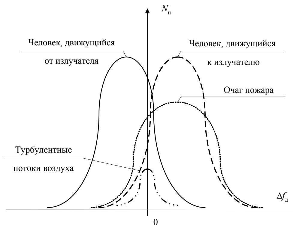
Рис. 5.1. Характерный вид спектра доплеровского сигнала для различных отражателей
