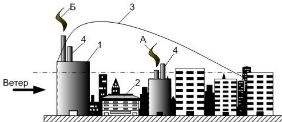
Рис. 1. Организация выброса загрязнений из низкого затененного здания:
